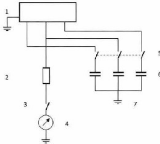
Hình 11. Sơ đồ mô phỏng thử nghiệm rò điện 1 pha
