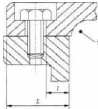
Hình 2. Mối ghép phòng nổ dạng ống, hình trụ có lỗ bắt bu lông
