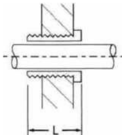
Hình 5. Mỗi ghép phòng nổ dạng trục xoay
