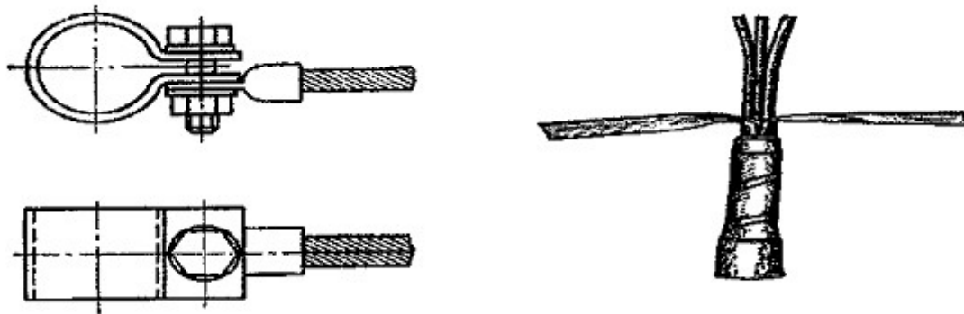
Hình 17 Phụ lục IV - Đai thép dùng để nối dây tiếp đất với vỏ chì và bằng thép cáp điện
