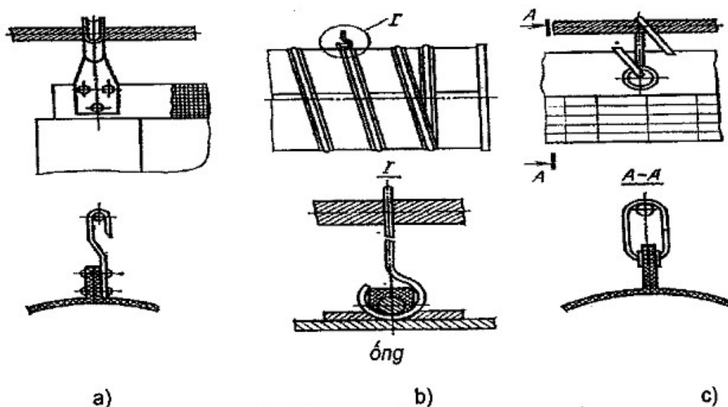
Hình 25 phụ lục IV - Tiếp đất các chi tiết kim loại của các ống thông gió mềm
