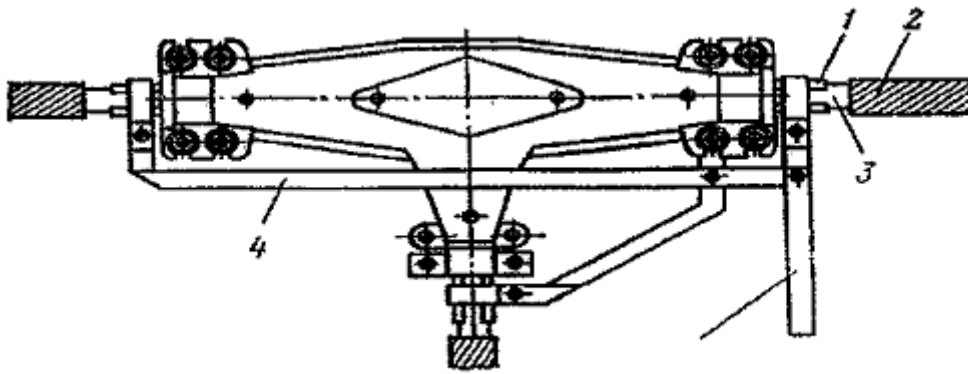
Hình 20 Phụ lục IV- Sơ đồ đầu tiếp đất cho múp chiếu sáng (múp nối 3 ngã)
