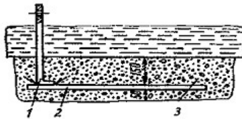
Hình 11 Phụ lục IV- Sơ đồ đặt vật tiếp đất trong lỗ khoan
