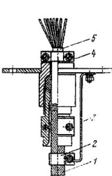
Hình 21 Phụ lục IV - Sơ đồ đầu tiếp đất cho cáp kiểm tra vỏ bọc chì
