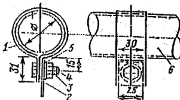
Hình 24 Phụ lục IV - Sơ đồ nối dây tiếp đất với các đường ống
