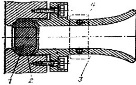
Hình 26 Phụ lục IV- Bịt kín lỗ cáp không sử dụng
