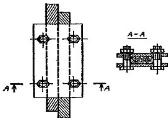
Hình 9 Phụ lục IV (b)- Sơ đồ xiết chặt dây tiếp đất trung gian với vít chống bê tông
