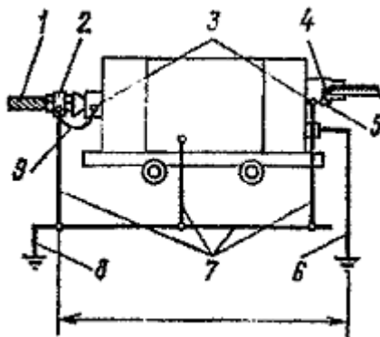
Hình 13 Phụ lục IV- Sơ đồ tiếp đất các trạm biến áp di động
