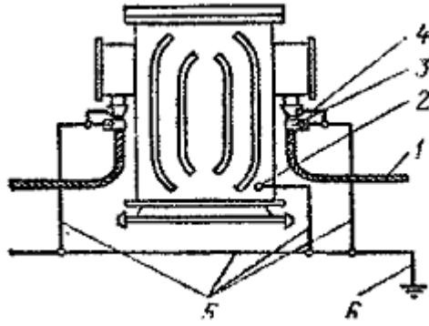
Hình 14 Phụ lục IV - Sơ đồ đấu tiếp đất các máy biến áp
