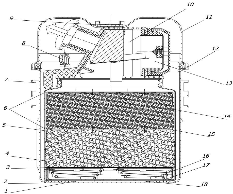
Hình 1 - Cấu tạo mẫu của bình tự cứu cá nhân dạng hấp thụ
