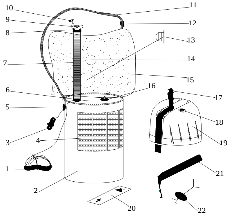
Hình 2 - Cấu tạo mẫu của bình tự cứu cá nhân dạng cách ly
