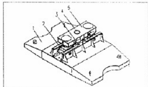
Hình A2.2.6 Cấu tạo cơ cấu di chuyển ngang và cụm bánh sắt di chuyển ngang: 1 - Chân di chuyển ngang; 2 - Cụm bánh sắt di chuyển ngang; 3 - Lò xo; 4 - Ổ trục quay trung tâm; 5 - Bàn quay.
