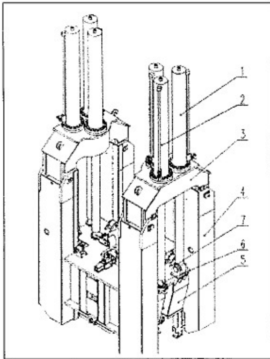
Hình A2.2.2 Cấu tạo của cơ cấu ép cọc: 1, 2 - Các xi lanh thủy lực ép cọc (chính và phụ); 3 - Dầm ngang đỡ các xi lanh thủy lực ép cọc; 4 - Trụ đứng dẫn hướng ép cọc; 5 - Hộp kẹp cọc; 6 - Ốc và chốt ghép cần của xi lanh thủy lực ép cọc với hộp kẹp cọc; 7 - Bát cầu trên hộp kẹp cọc 5 có nhiệm vụ tiếp nhận đầu dạng cầu tròn của các xi lanh thủy lực ép cọc phụ
