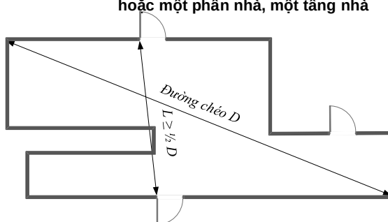
b) Minh họa về bố trí phân tán lối ra thoát nạn của các gian phòng nằm trong một gian phòng khác hoặc một phân nhà, một tầng nhà
