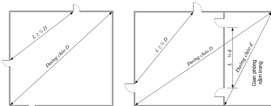
a) Minh họa về bố trí phân tán lối ra thoát nạn của một gian phòng, một phân nhà hoặc một tầng nhà
