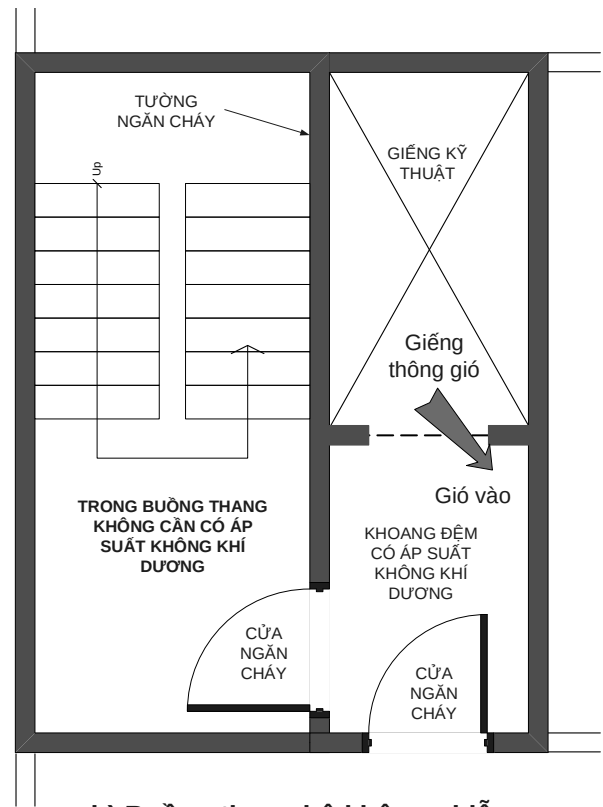
b) Buồng thang bộ không nhiễm khói loại N3
