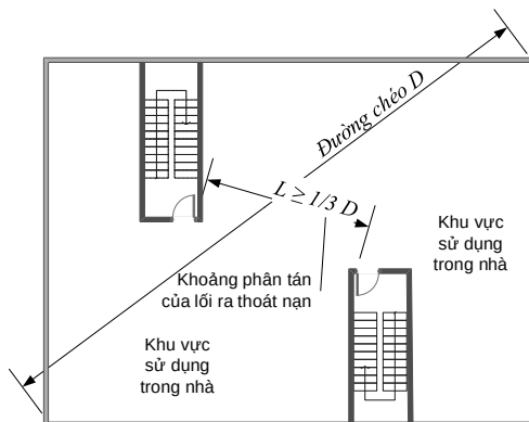
d) Trường hợp toàn nhà được bảo vệ bằng hệ thống sprinkler, có thể giảm khoảng phân tán của lối ra thoát nạn L D
