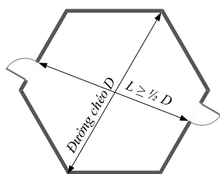
a) Minh họa về bố trí phân tán lối ra thoát nạn của một gian phòng, một phân nhà hoặc một tầng nhà
